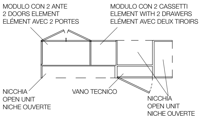
VISTA DALL'ALTO/SEZIONE TOP VISION/SECTION VUE DE DESSUS/SECTION
