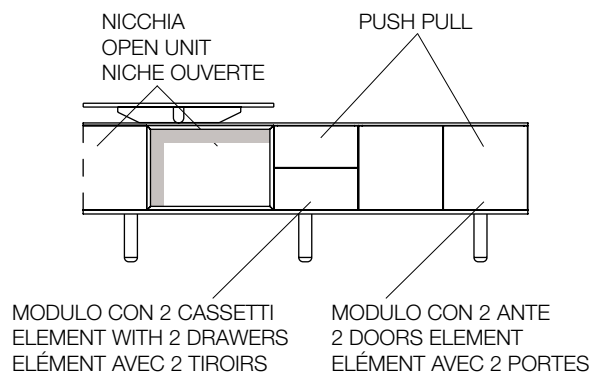
VISTA LATERALE - LATO UTENTE SIDE VISION - USER SIDE VUE CÔTÉ OPÉRATEUR
